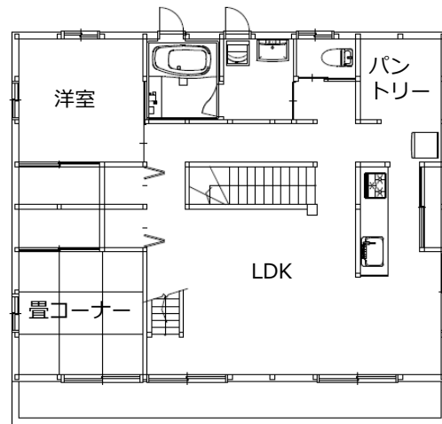
2F 施工面積 80,00㎡ (24,2坪)
