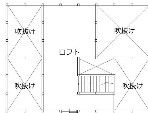
ロフト 施工面積 18,00㎡ (5,4坪)
